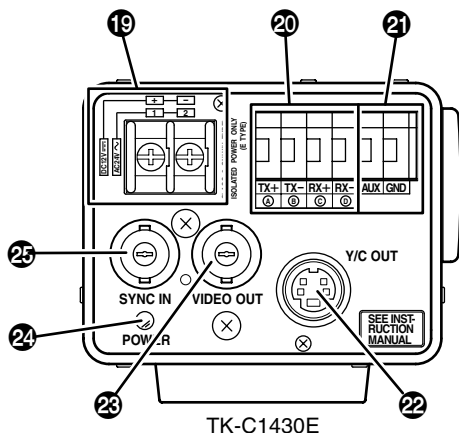
TK-C1430E
